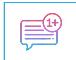
Get Message
